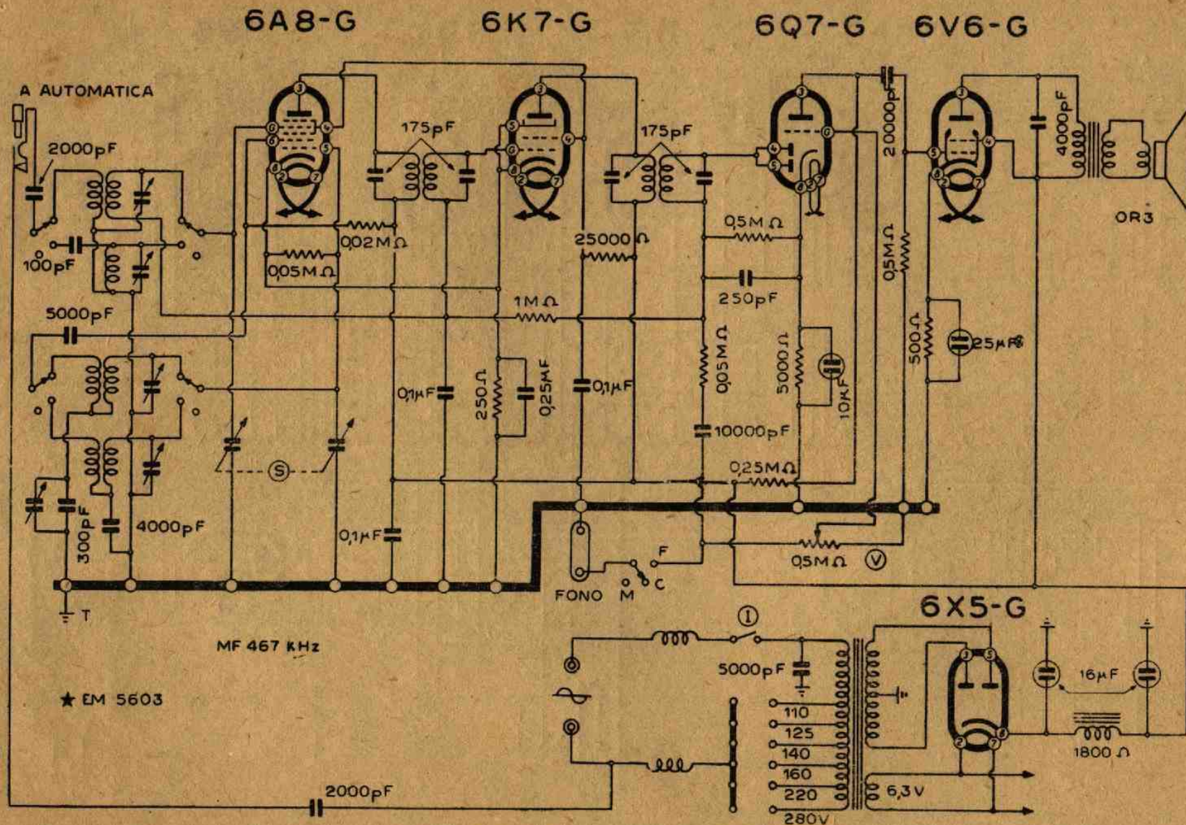
Lo schema elettrico del mod. 522
